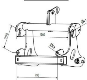
Anbauseite Lader
