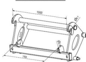
Laderseite Euro Norm
