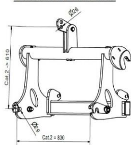
Anbauseite 3-Pkt Laster
