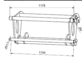
Werkzeugseite HauerB mech. Verriegelung
