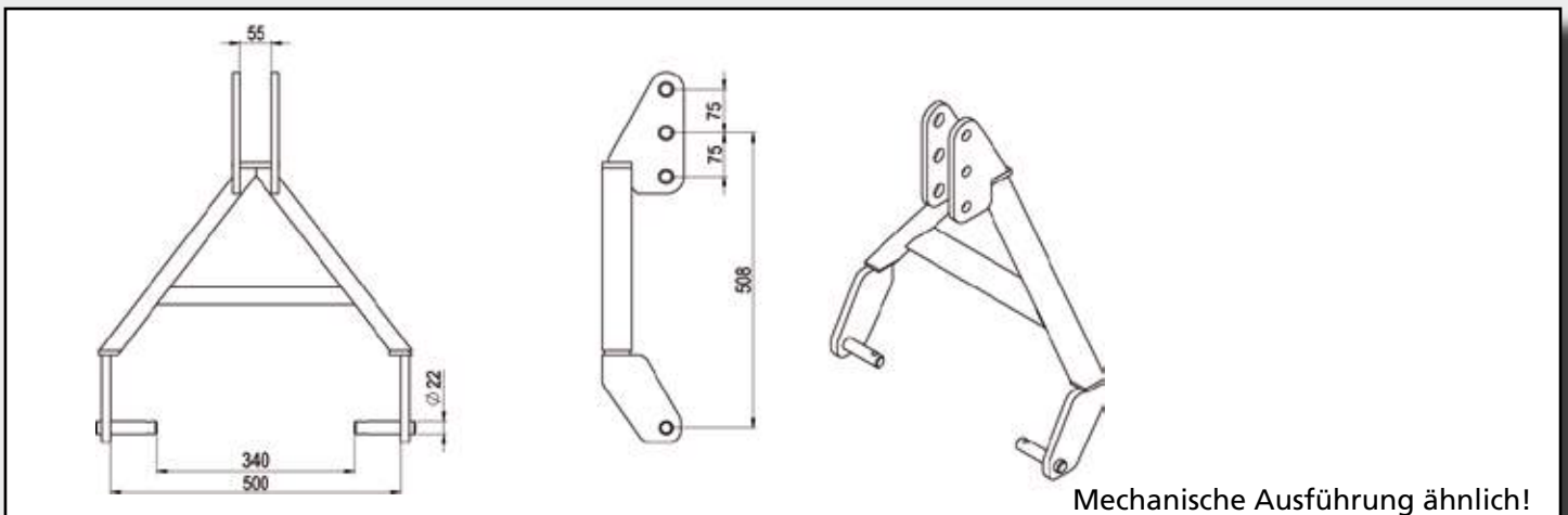
Dreipunktbock: KAT I N
