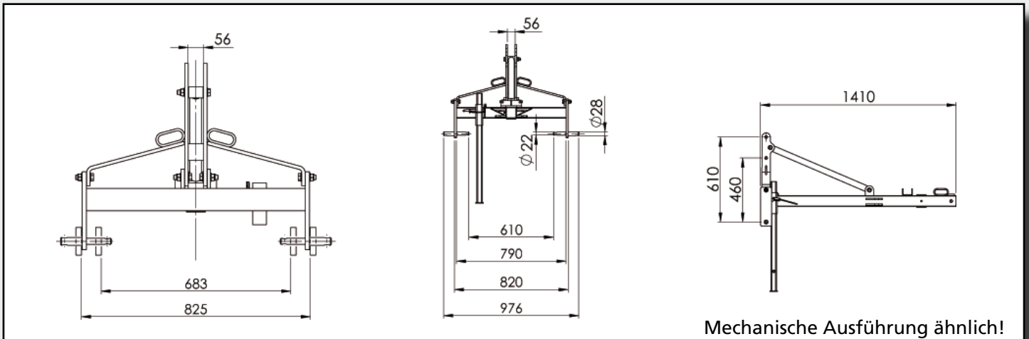
Dreipunktbock: KAT I / II
