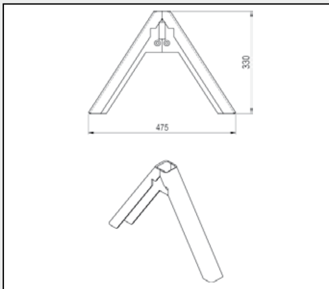
Gerätedreieck: KAT Kommunal
